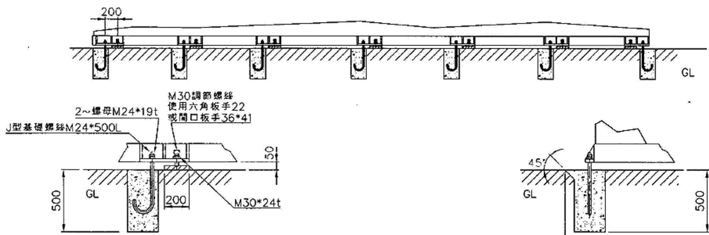
SECTION A-A
